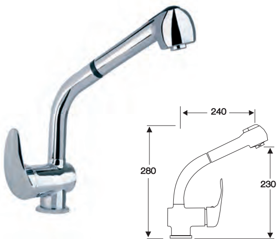
SERIE OMEGA "extraible" Cromo Ref. 24007
